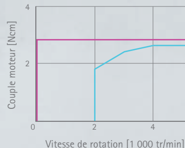
Courbe caractéristique du moteur
