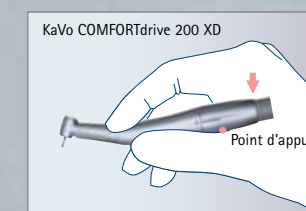
L'équilibre parfait pour un travail confortable : la zone lourde derrière le point d'appui de l'instrument est considérablement réduite pour le KaVo COMFORTdrive. L'effort nécessaire pendant le travail est sensiblement réduit.
